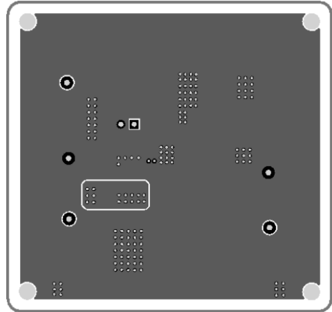
Fig. 17 Bottom Layer
