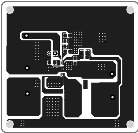
Fig. 16 Top Layer
